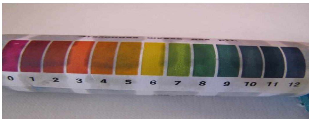
Рисунок 2. Определение pH
